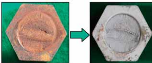
写真2 破面錆除去
