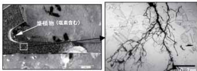
写真4 断面でのき裂形状(ステンレス鋼 応力腐食割れ)
