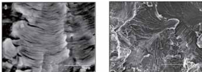
ストライエーション(疲労破壊) 流れ模様(応力腐食割れ) 写真3 ミクロフラクトグラフィ(SEM観察)
