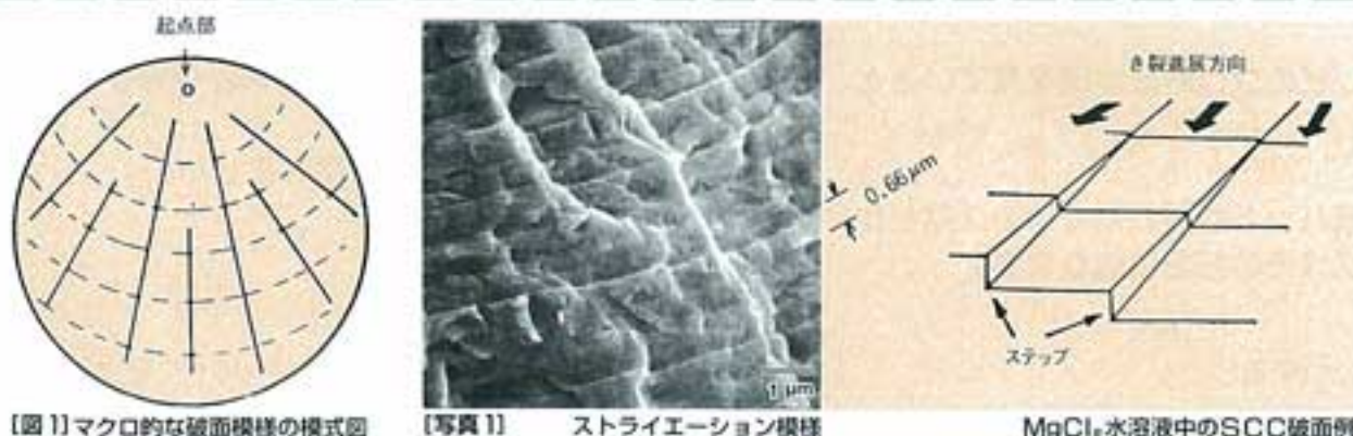
[図1] マクロ的な破面模様の模式図 [写真1] ストライエーション模様 MgCl 2 水溶液中のSCC破面例
