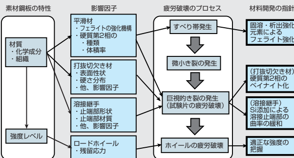
図1 ●高疲労強度ホイール用鋼板開発のための研究内容
