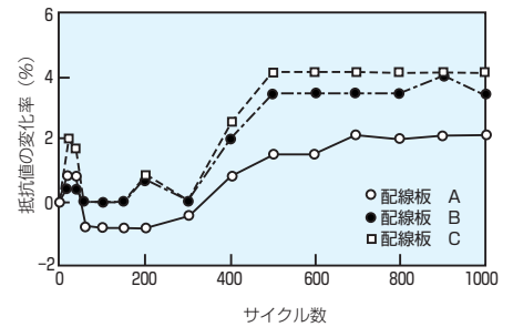
図1 ●熱衝撃試験の抵抗値変化例 (スルーホールチェーン)
