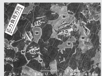
写真2 ●マルテンサイト(M)間のフェライト(黒色部)に発生したすべり帯(sb)(SEM観察)
