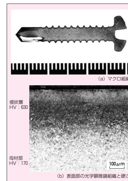
【写真3】ドリルねじ
