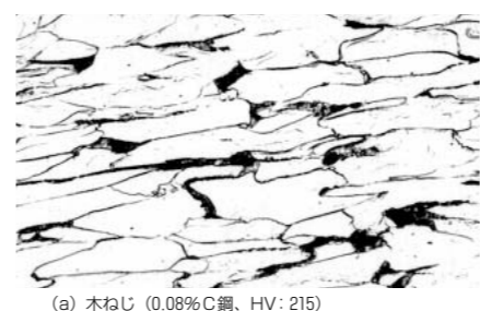
(a) 木ねじ (0.08% C鋼, HV: 215)
