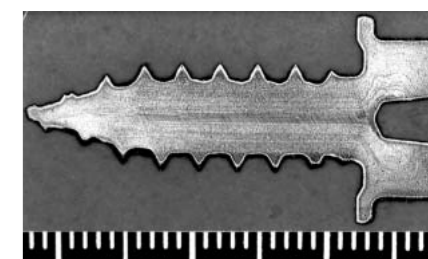
【写真4】六角フランジ付きタッピングねじのマクロ組織
