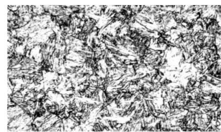
(b) タッピングねじ (0.24% C鋼, HV: 392)
