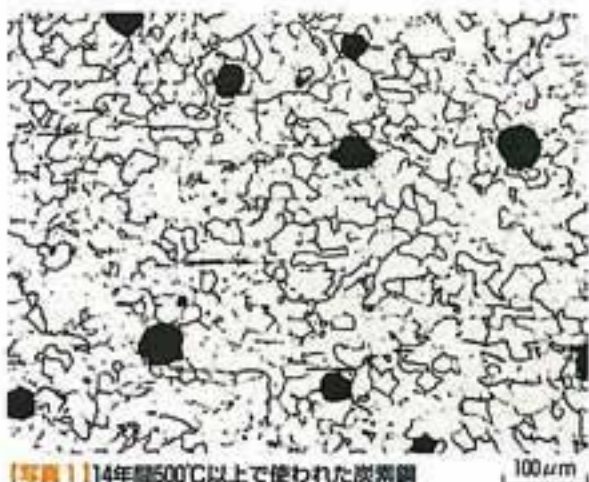
【写真1】14年間500°C以上で使われた炭素鋼
