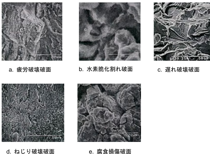
【写真3】各種破壊破面のSEM像
