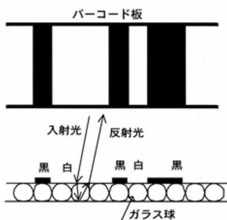
図2 再帰性バーコードの模式図
