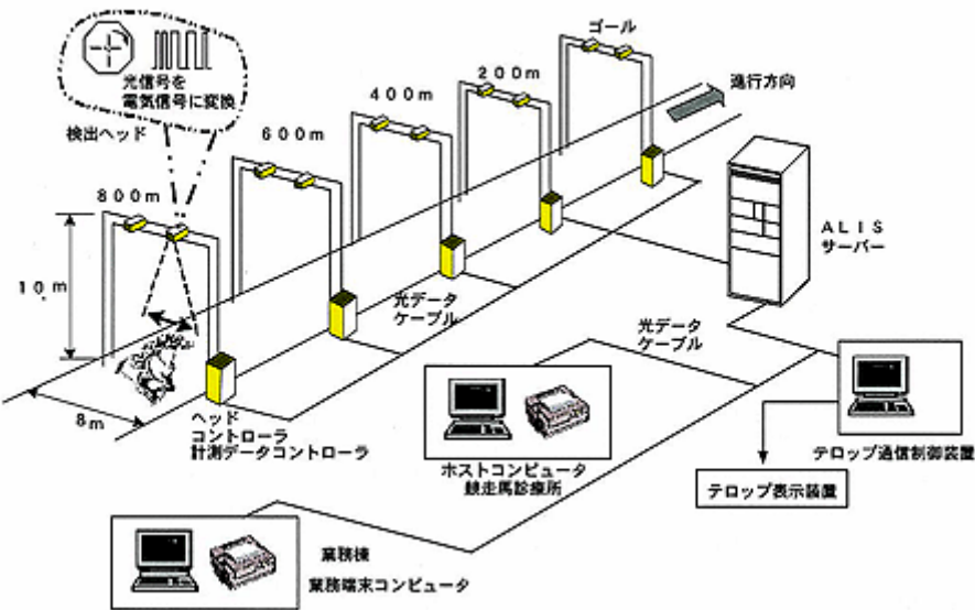
図1 ALIS システムの概要図
